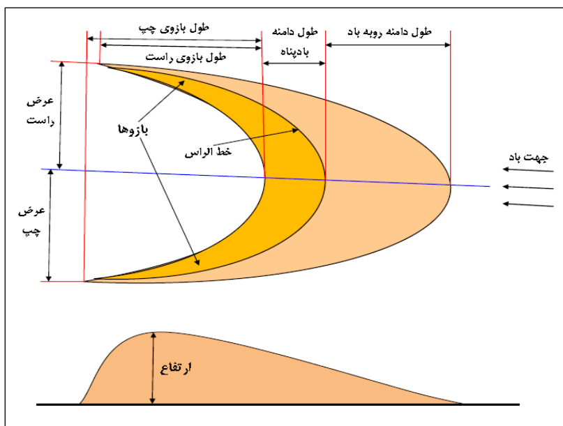
شکل (۴): مهم‌ترین مولفه‌های مورفومتری برخان و مدل اندازه‌گیری آن‌ها: ارتفاع (H)؛ عرض پهلوئی راست (W a )؛ عرض پهلوئی چپ (W b )؛ طول بازوی راست (L a )؛ طول بازوی چپ (L b )؛ طول دامنه ی روبه‌باد (L 0 )؛ طول دامنه‌ی بادپناه (L S ).
