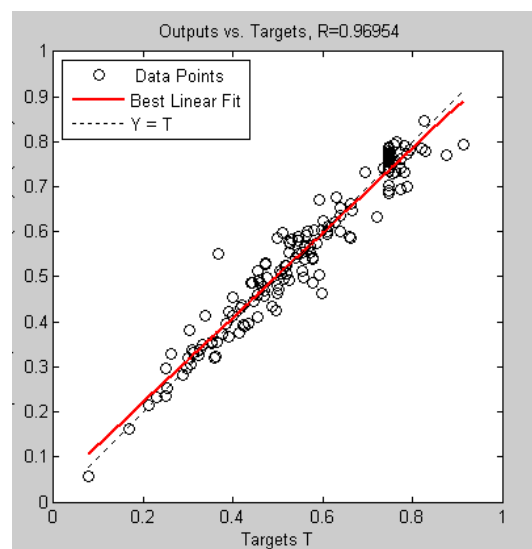
شکل ۴- ضرایب همبستگی مدل شماره ۱ (الگوریتم پس انتشار) در مرحله آموزش و تست. (الف، ب) ضرایب همبستگی به ترتیب در مرحله آموزش و آزمایش
