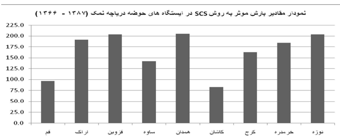
▲ شکل ۲) نمودار بارش مؤثر سالانه ایستگاه‌های حوضه دریایچه نمک بر اساس روش SCS (۱۳۸۷ - ۱۳۶۶)
