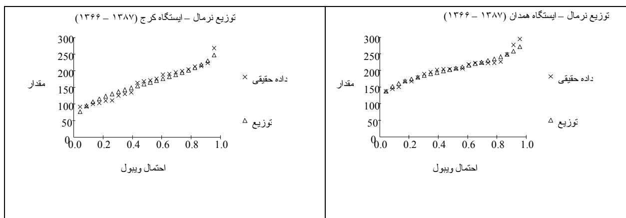
▲ شکل ۴) برازش داده های مقادیر بارش مؤثر ماهانه دو ایستگاه حوضی دریاچهی نمک با توابع توزیع احتمالات مختلف (۱۳۶۶ - ۱۳۸۷)
