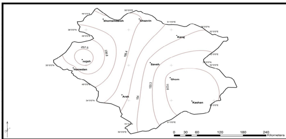
▲ شکل ۱) موقعیت جغرافیایی و نقشه همبارش مؤثر سالانه حوضه دریایچه نمک (۱۳۸۷ - ۱۳۶۶)
