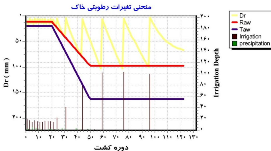
شکل ۱۰: منحنی تغییرات رطوبت خاک در دشت سبزواری
