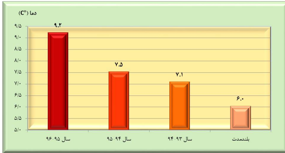
شکل ۶: تغییرات میانگین دمای فصل پاییز در ایستگاه کوهرنگ نسبت به بلندمدت (درجه‌ی سانتی‌گراد)
