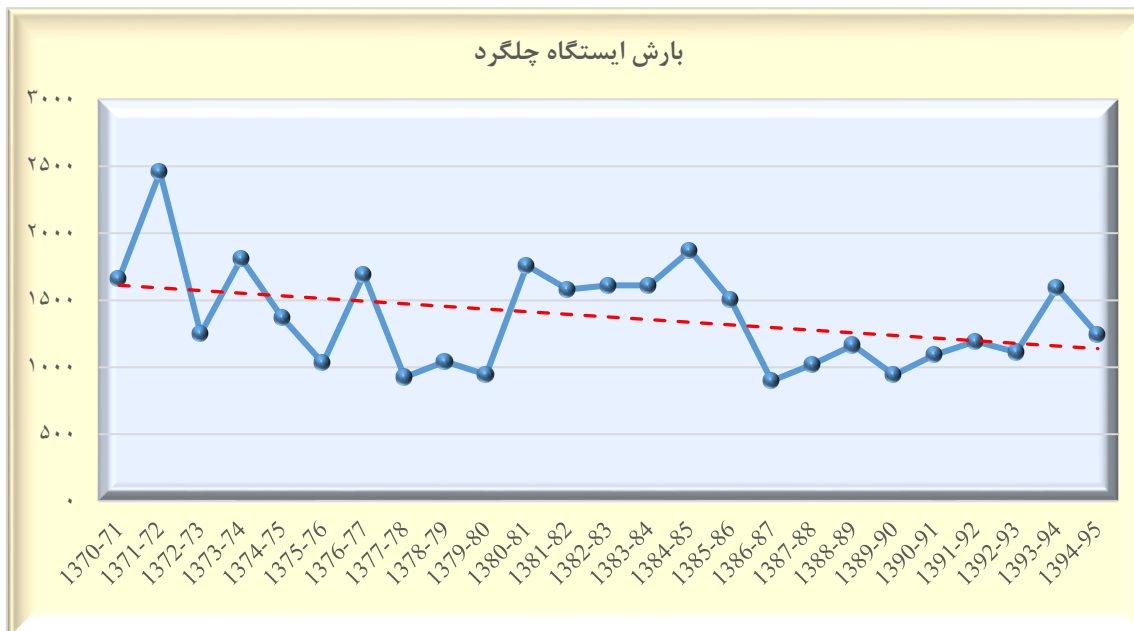
شکل ۴: تغییرات سالیانه بارش در ایستگاه چلگرد در دوره ۲۵ ساله (۱۳۹۵-۱۳۷۰) - میلی متر
