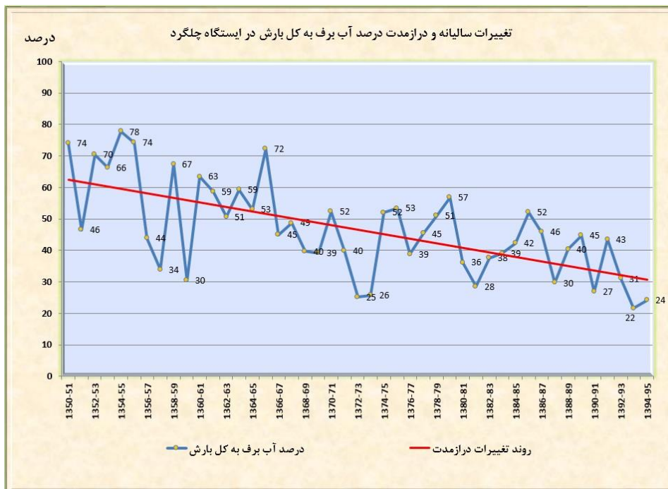
شکل ۷: میزان سالانه درصد آب برف به کل بارش در ایستگاه چلگرد (۱۳۵۰-۹۵)
