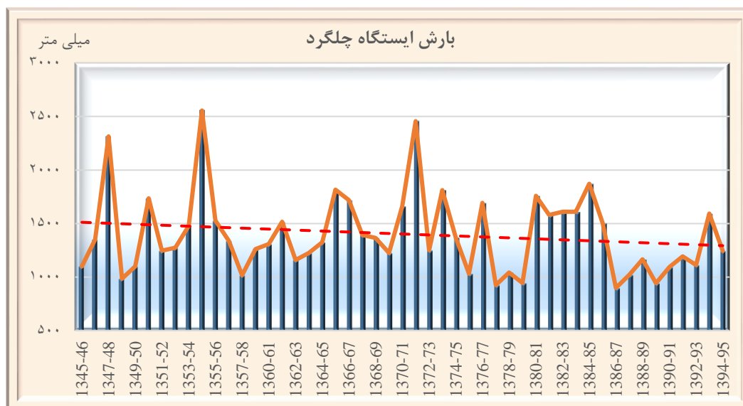
شکل ۳: تغییرات سالیانه بارش در ایستگاه چلگرد در دوره ۵۰ ساله (۱۳۹۵-۱۳۴۵) - میلی متر
