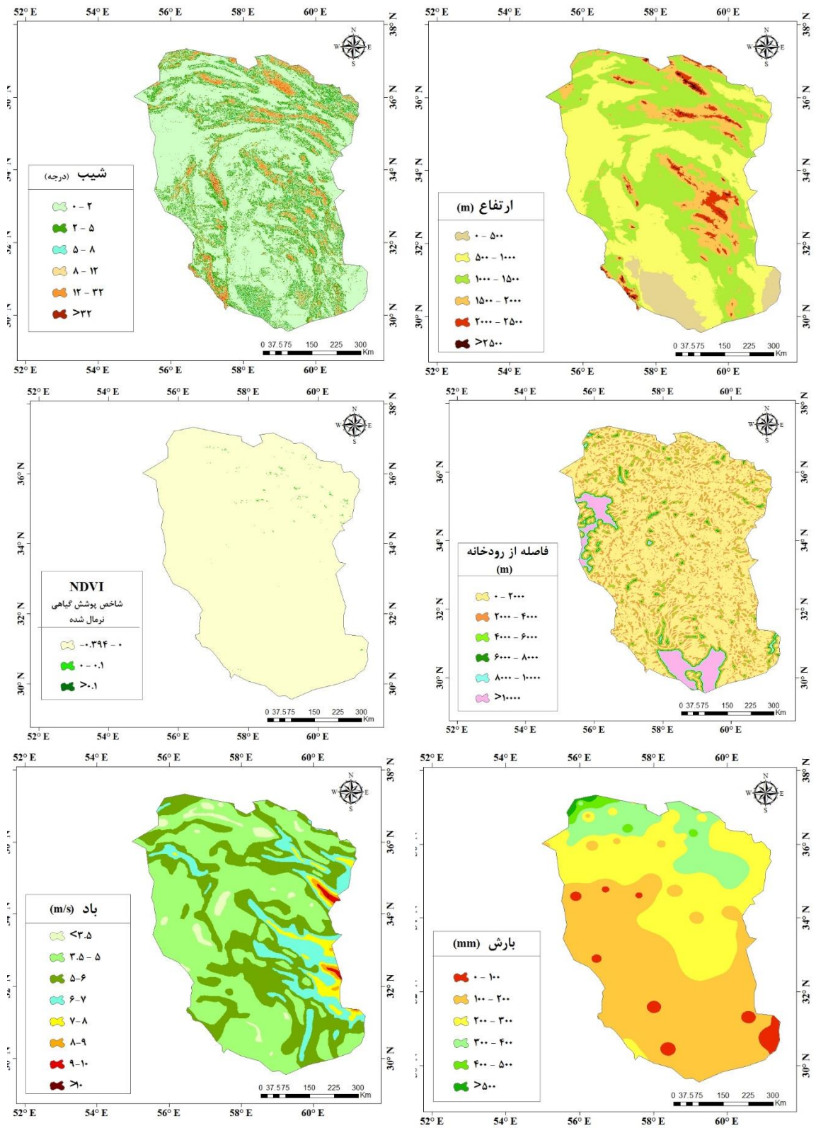
شکل ۲: نقشه‌ی عوامل مؤثر بر مناطق برداشت گردوغبار در منطقه‌ی مورد مطالعه
