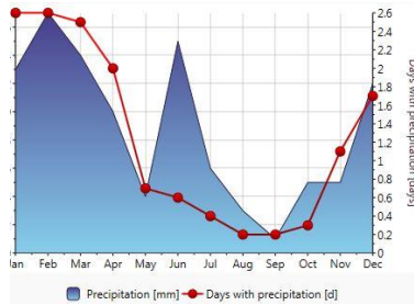
شکل ۱۵: وضعیت بارش ماهانه
