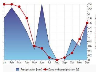
شکل ۹: وضعیت بارش ماهانه
