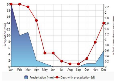
شکل ۳۳: وضعیت بارش ماهانه
