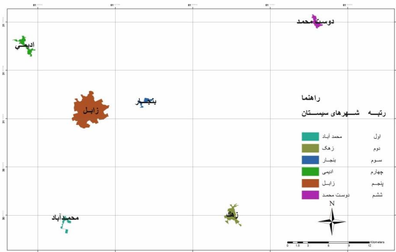
شکل ۴۰: پهنه‌بندی نهایی منطقه‌ی مورد مطالعه
