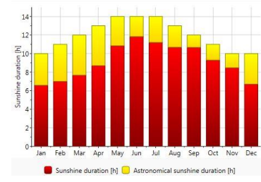
شکل ۳۵: وضعیت مدت تابش
