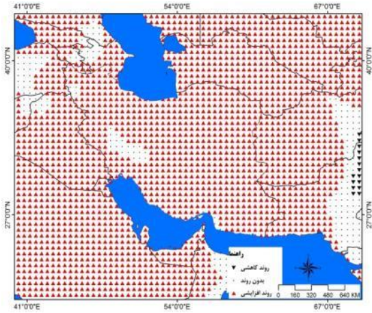
شکل ۲۰: روند دمایی کمینه‌ی ماه اوت
