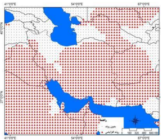
شکل ۵: روند دمای بیشینه‌ی ماه می
