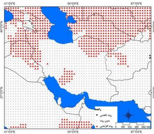
شکل ۳: روند دمای بیشینه‌ی ماه مارس
