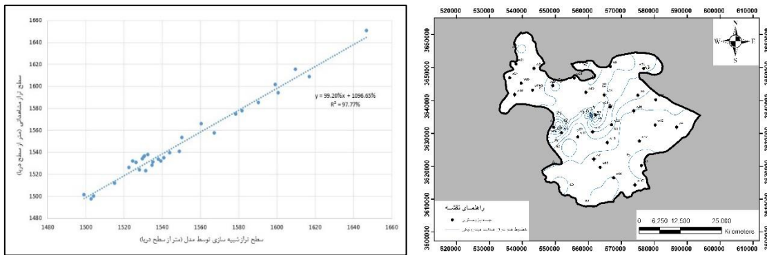
شکل ۶: نمودار سطح تراز ایستایی مشاهده‌ای و شبیه‌سازی شده و هدایت هیدرولیکی بهینه‌سازی شده‌ی آبخوان
