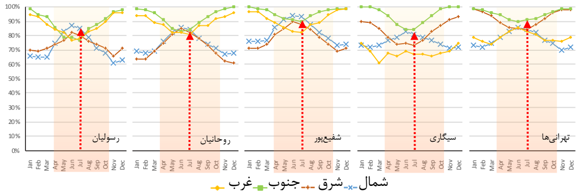
شکل ۱: میانگین سایه‌اندازی جداره‌های حیاط‌های مرکزی مورد مطالعه (برحسب درصد)
