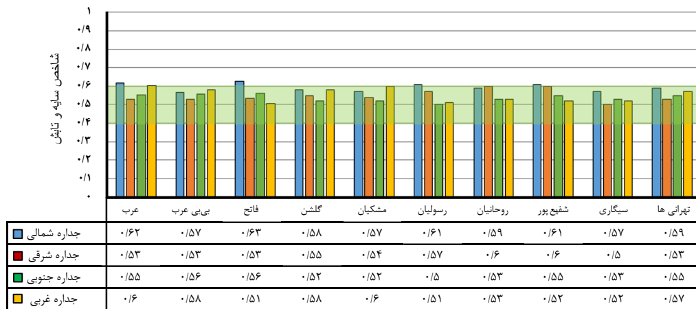
شکل ۵: شاخص سایه-تابش سالیانه‌ی جداره‌های حیاط‌های مرکزی
